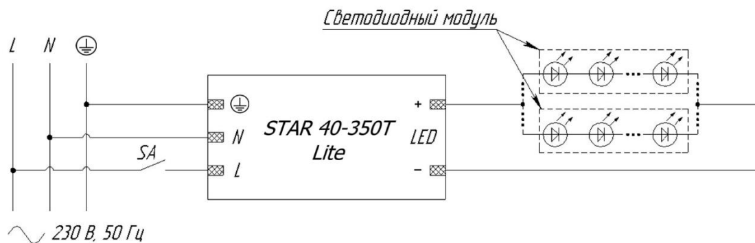
а) Схема параллельного соединения светодиодных модулей
